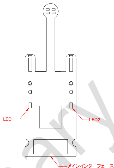
インターフェース配置図
